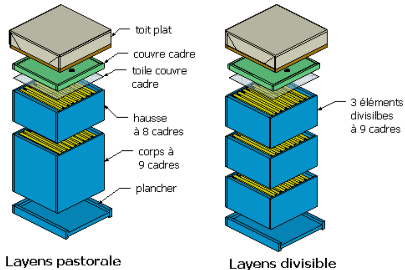
Fig. 1 : Schéma de deux modèles de ruche
